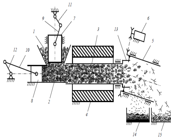
Рис. 1. Принципиальная схема установки для отделения хвои СВЧ-нагревом
