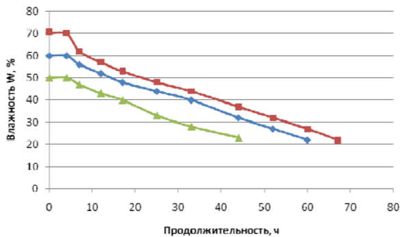
Рис. 4. Кривые сушки шпалы из древесины березы от начальной влажности 70 %, 60 % и 50 % до конечной 22 % при температуре среды 130 °С
