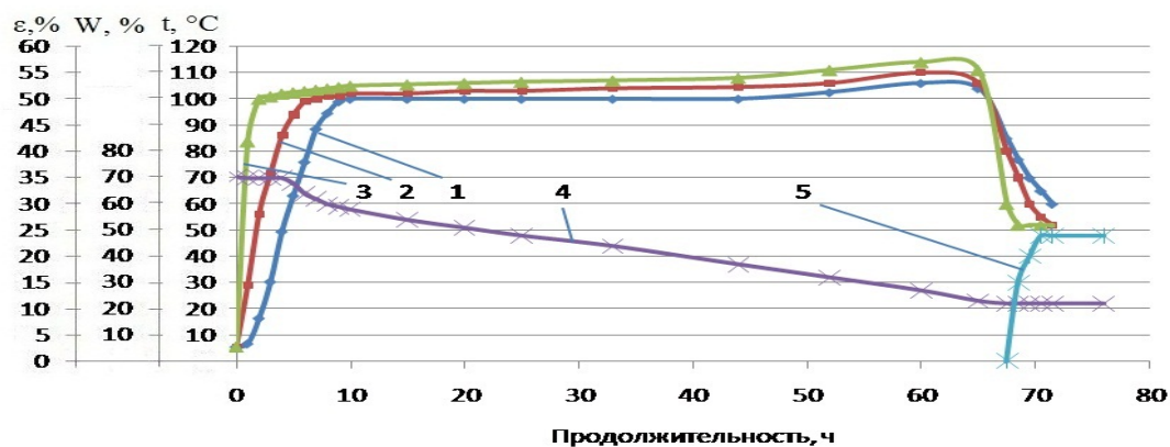
1, 2, 3 – температура (t) в центре заготовки, на расстоянии 0,5R (радиуса) и 0,25R (радиуса); 4 – кривая влажности (W); 5 – степень прессования заготовки (ε)
