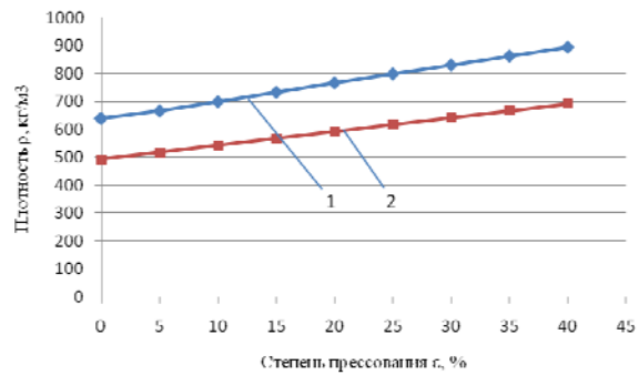
Рис. 1. Зависимость плотности древесины березы и осины от степени прессования
