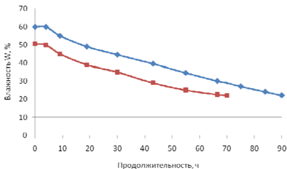
Рис. 5. Кривая сушки шпалы из древесины березы от начальной влажности 60 % и 50 % до конечной 22 % при температуре среды 120 °С
