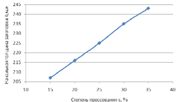
Рис. 2. Зависимость начального размера заготовки по толщине от степени прессования
