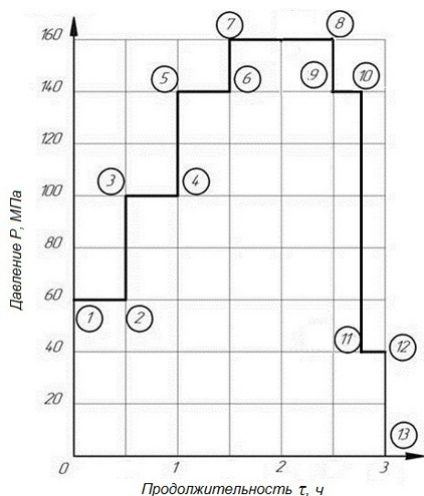
Рис. 6. Циклограмма давления при операции прессования
