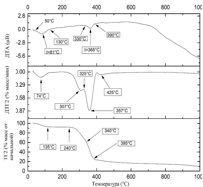
Рис. 4. Комплексная термограмма багассы в защитной среде
