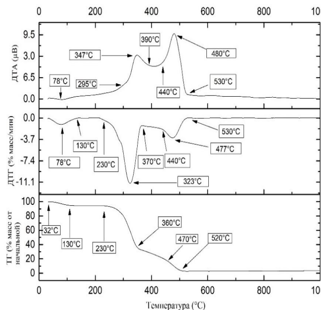
Рис. 2. Комплексная термограмма багассы в окислительной среде
