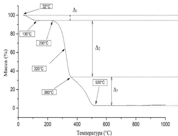
Рис. 3. Термогравиметрическая кривая багассы в окислительной атмосфере
